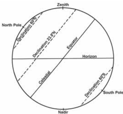
Figure 1316c. The oblique sphere at latitude 40^\circ\text{N} .
